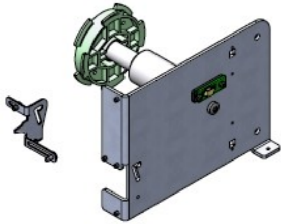
Papierrollenhalter mit Papieranschlag
